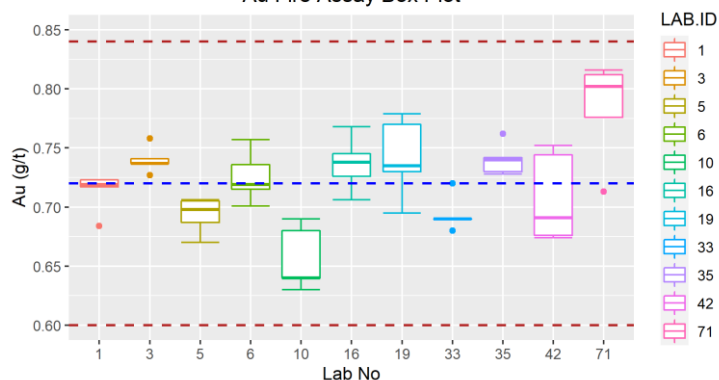
Au Fire Assay Box Plot
