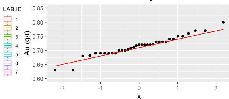
Au Photon Assay Q-Q Plot
