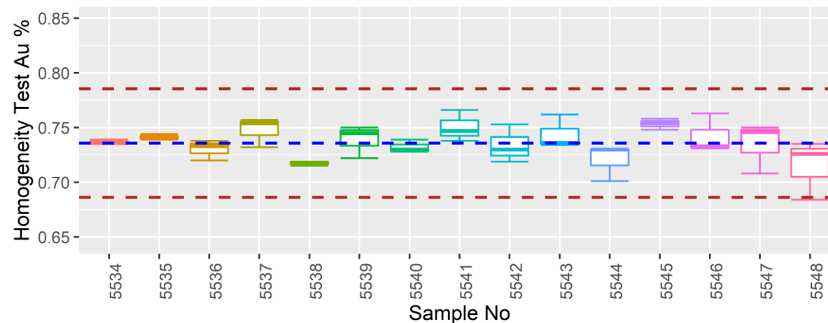
Au Fire Assay Box Plot
