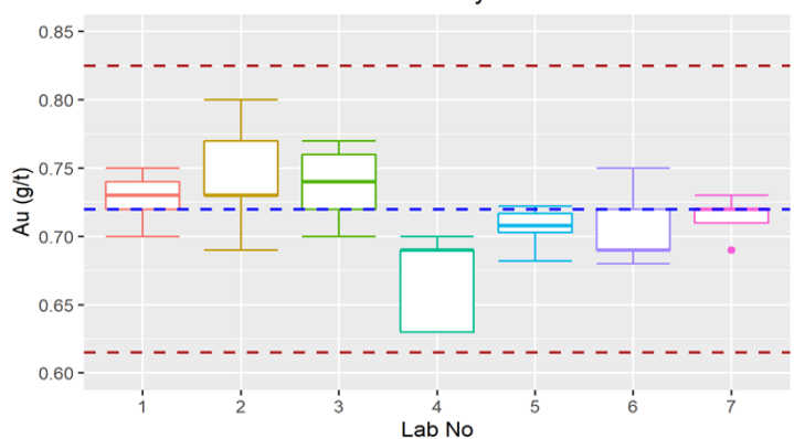
Au Photon Assay Box Plot
